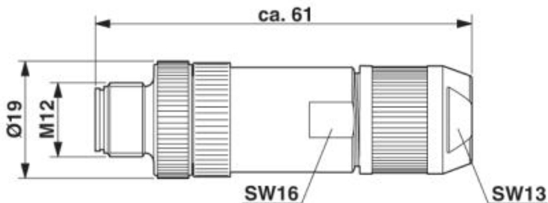
尺寸图
